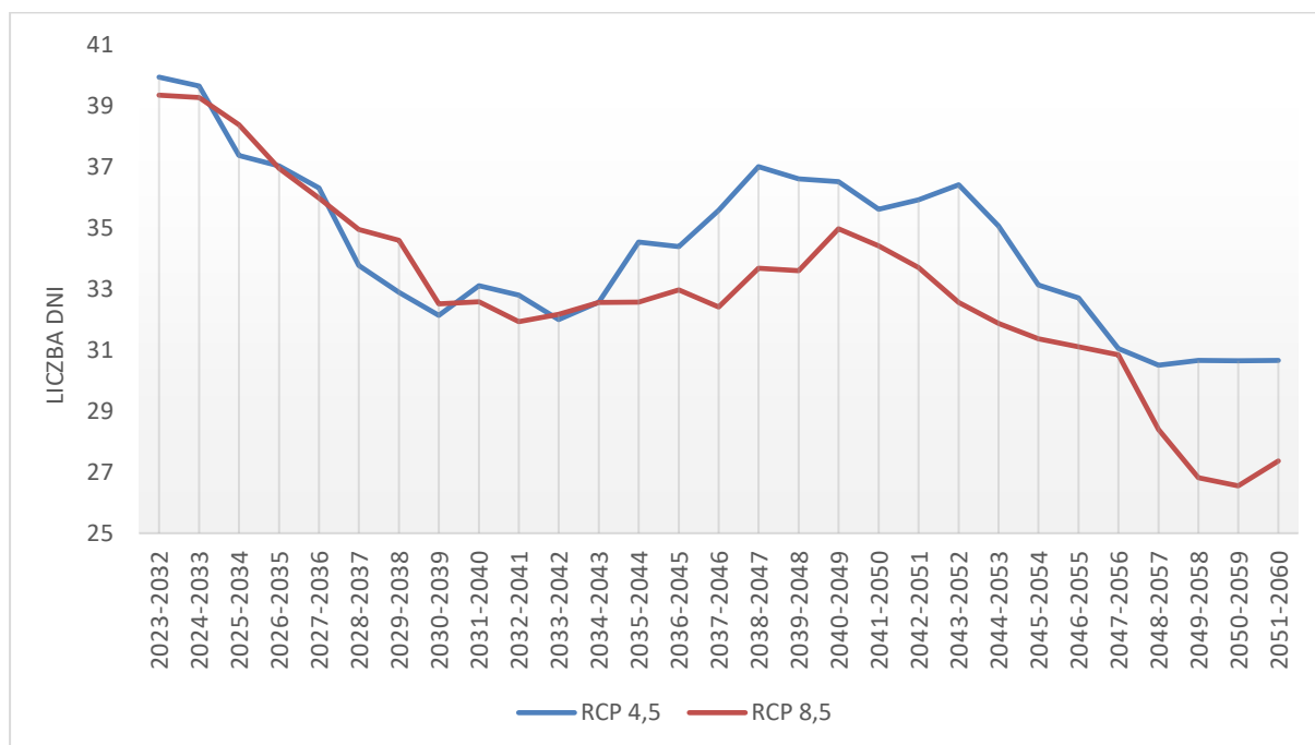
Rysunek 61 Średnia krocząca liczby dni mroźnych ( T_{max} < 0^{\circ}C ) do 2060 roku (w podziale na dekady) na obszarze powiatu sokólskiego według scenariusza RCP 4.5 i 8.5 (źródło: opracowanie własne na podstawie danych projekcji klimatycznych dla Polski, KLIMADA 2.0, https://klimada2.ios.gov.pl/klimat-scenariusze-portal/ )
