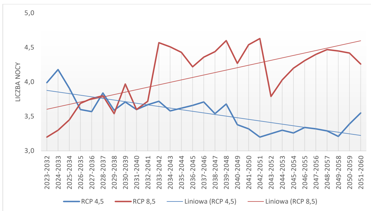
Rysunek 64 Średnia krocząca liczby nocy tropikalnych ( T_{min} > 20^{\circ}\text{C} ) do 2060 roku (w podziale na dekady) na obszarze powiatu sokólskiego według scenariusza RCP 4.5 i 8.5 (źródło: opracowanie własne na podstawie danych projekcji klimatycznych dla Polski, KLIMADA 2.0, https://klimada2.ios.gov.pl/klimat-scenariusze-portal/ )
