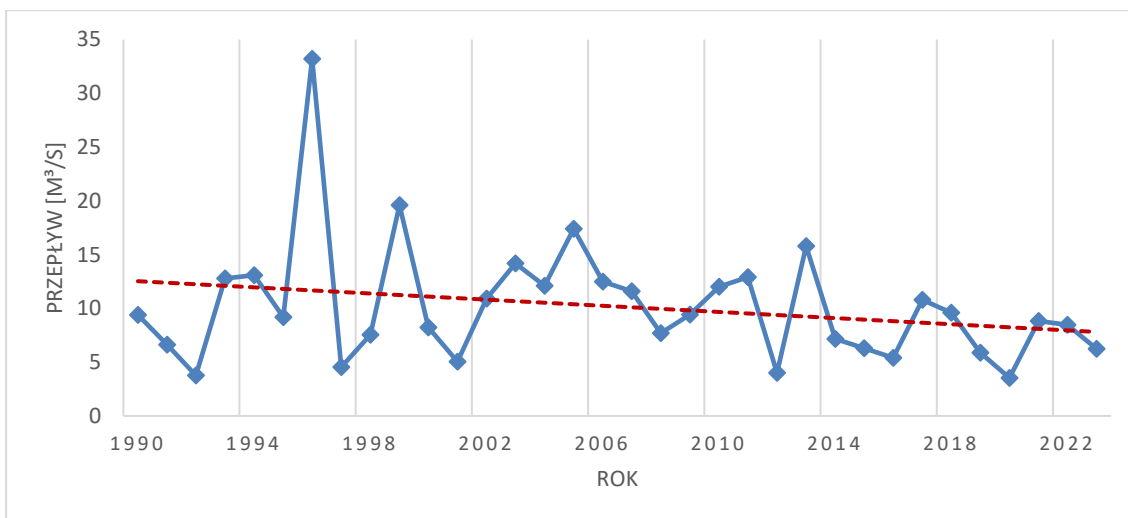
Rysunek 53 Średnioroczny przepływ maksymalny [ \text{m}^3/\text{s} ] w latach 1990-2023 (stacja Sokołda) (źródło: opracowanie własne na podstawie danych IMGW-PIB)
