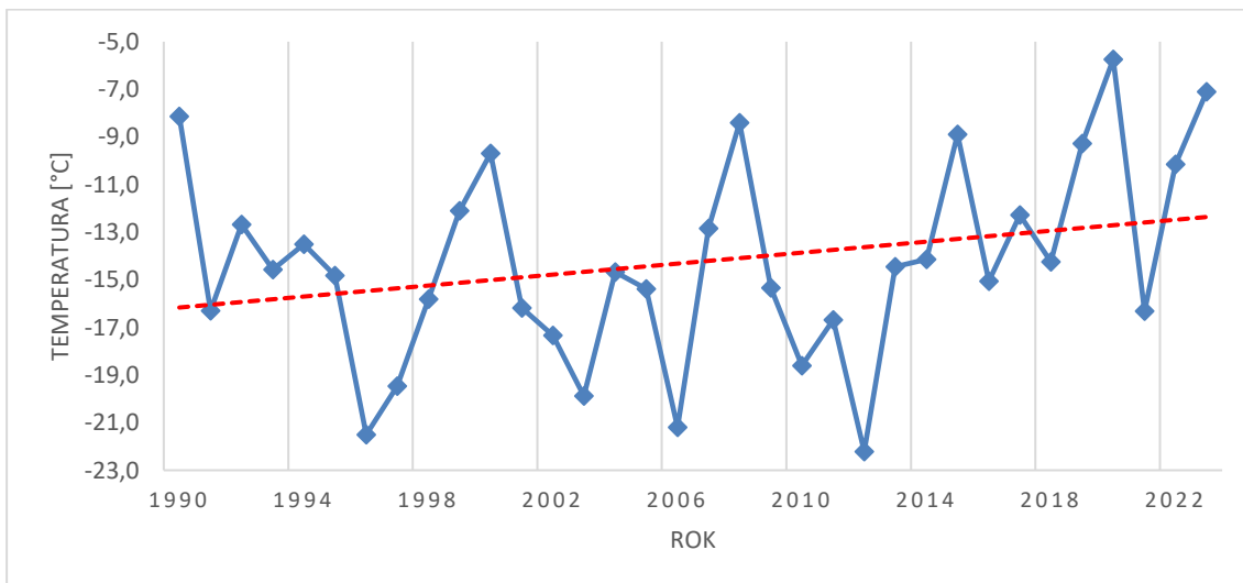
Rysunek 18 Percentyl 2% temperatury minimalnej powietrza [ ^{\circ}\text{C} ] w latach 1990-2023 (stacja Białystok) (źródło: opracowanie własne na podstawie danych IMGW-PIB)
