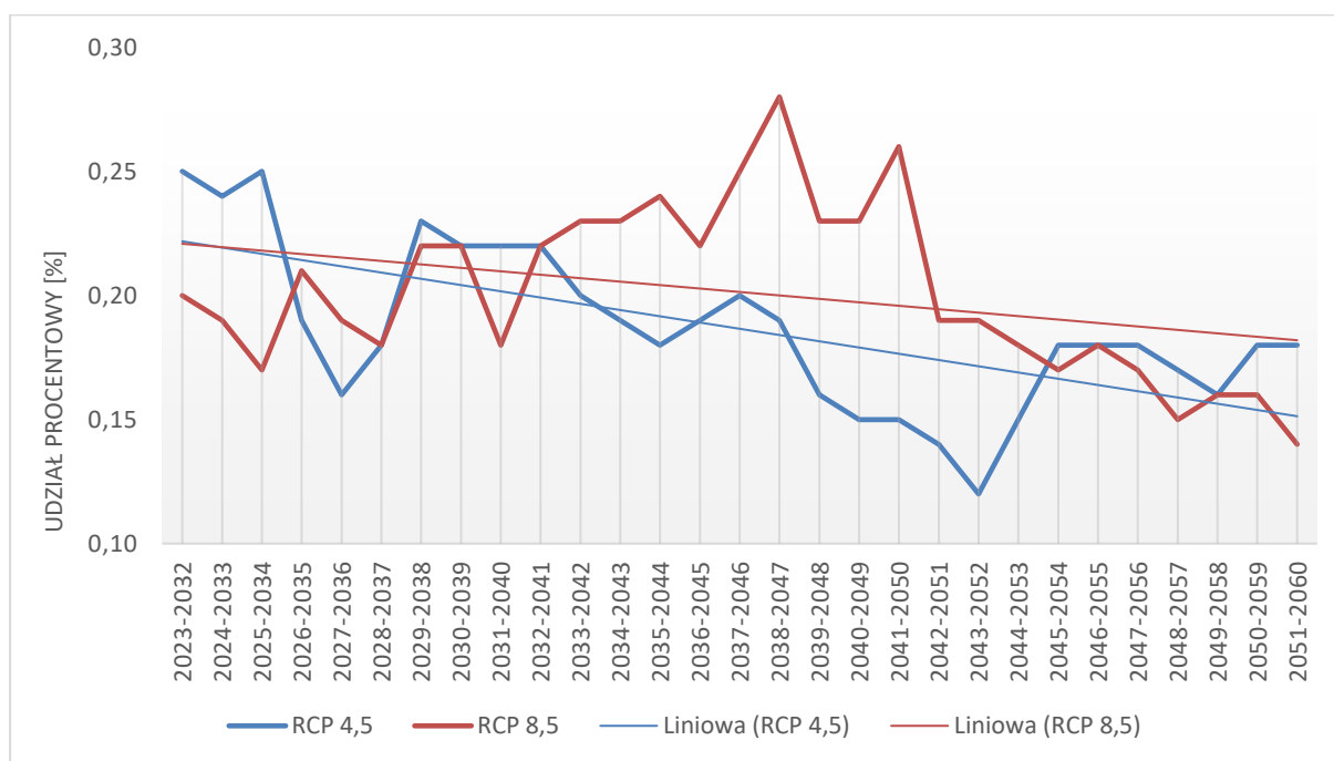
Rysunek 76 Średnia krocząca średniego udziału wiatrów silnych i bardzo silnych [10-30 m/s] do 2060 roku (w podziale na dekady) na obszarze powiatu sokólskiego według scenariusza RCP 4.5 i 8.5 (źródło: opracowanie własne na podstawie danych projekcji klimatycznych dla Polski, KLIMADA 2.0, https://klimada2.ios.gov.pl/klimat-scenariusze-portal/ )
