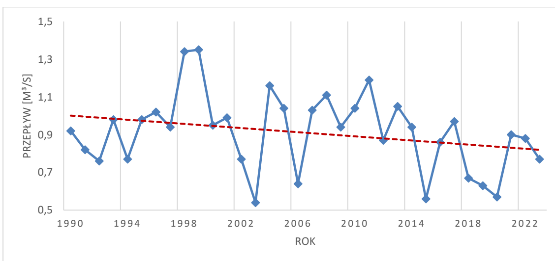
Rysunek 54 Średnioroczny przepływ minimalny [ \text{m}^3/\text{s} ] w latach 1990-2023 (stacja Sokołda) (źródło: opracowanie własne na podstawie danych IMGW-PIB)
